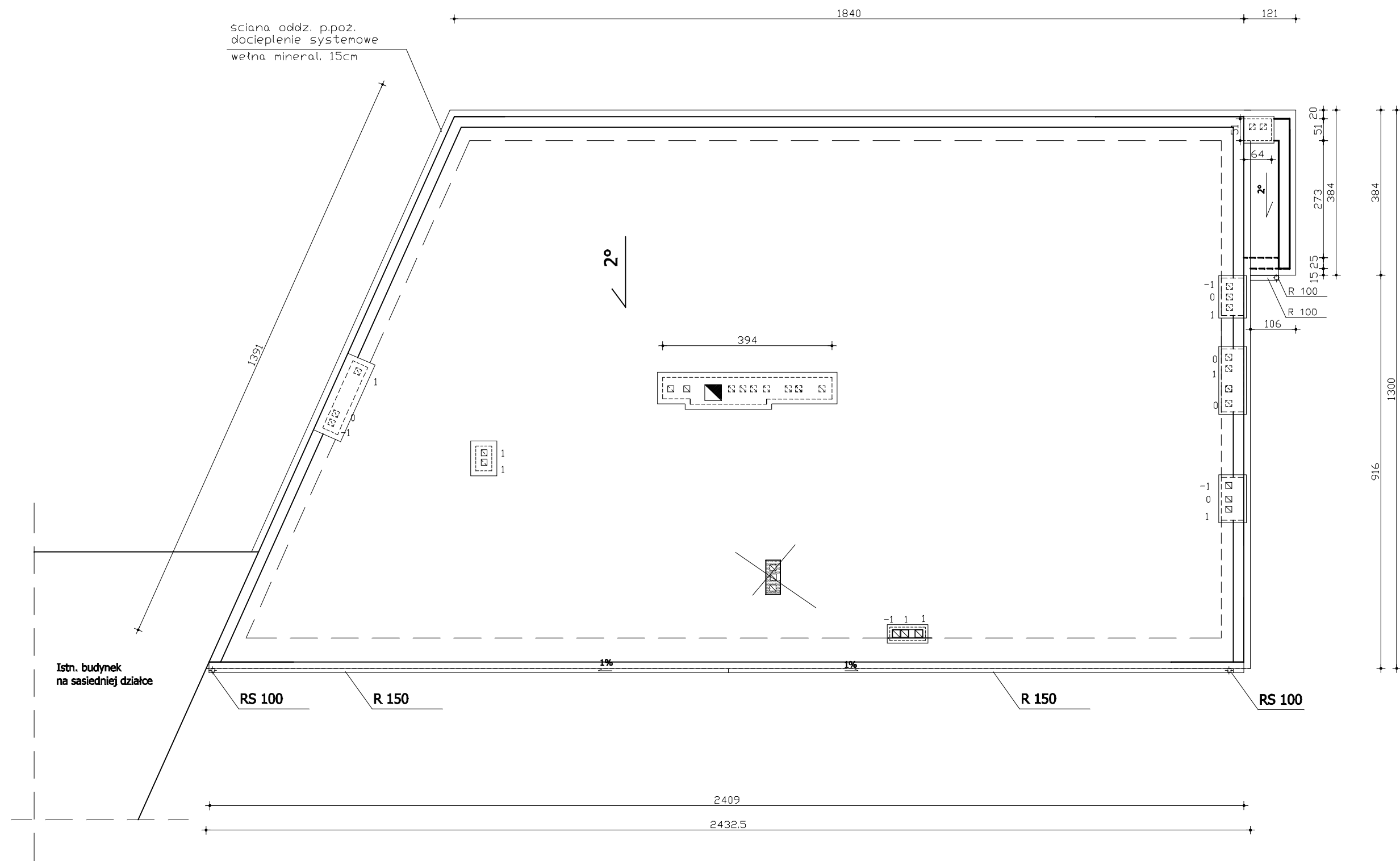
RZUT DACHU Skala 1 : 100
